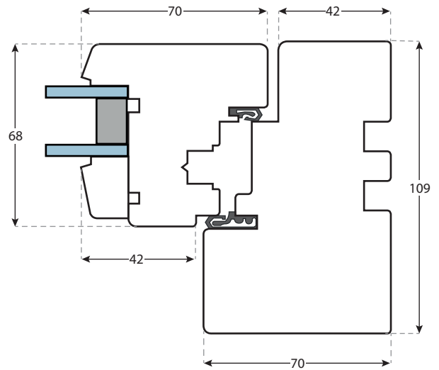
Stulp für zweiflügelige Elemente ohne Setzholz mit beidseitiger Schlagleiste
