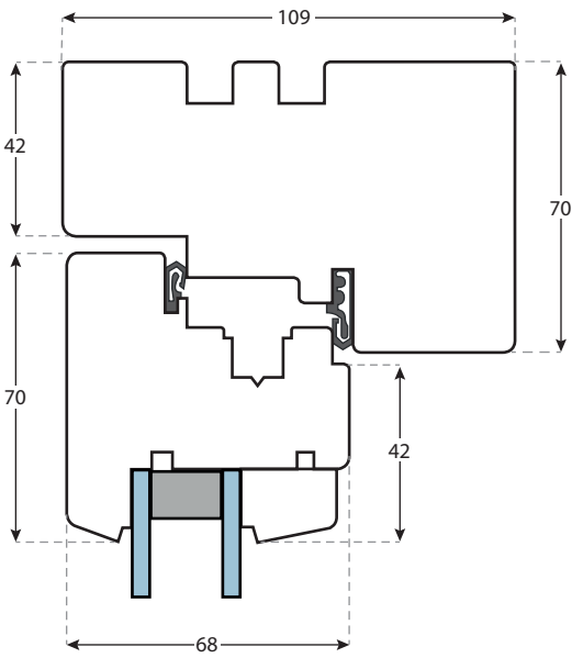
Kämpfer für Elemente mit Oberlicht
